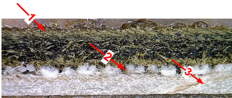
Рис. 2 Поперечный срез материалов обуви: 1 – кожевенные волокна верха обуви, 2 – прокладка – трикотажное полотно (хлопок – 100%), 3 – кожевенные волокна подкладки
